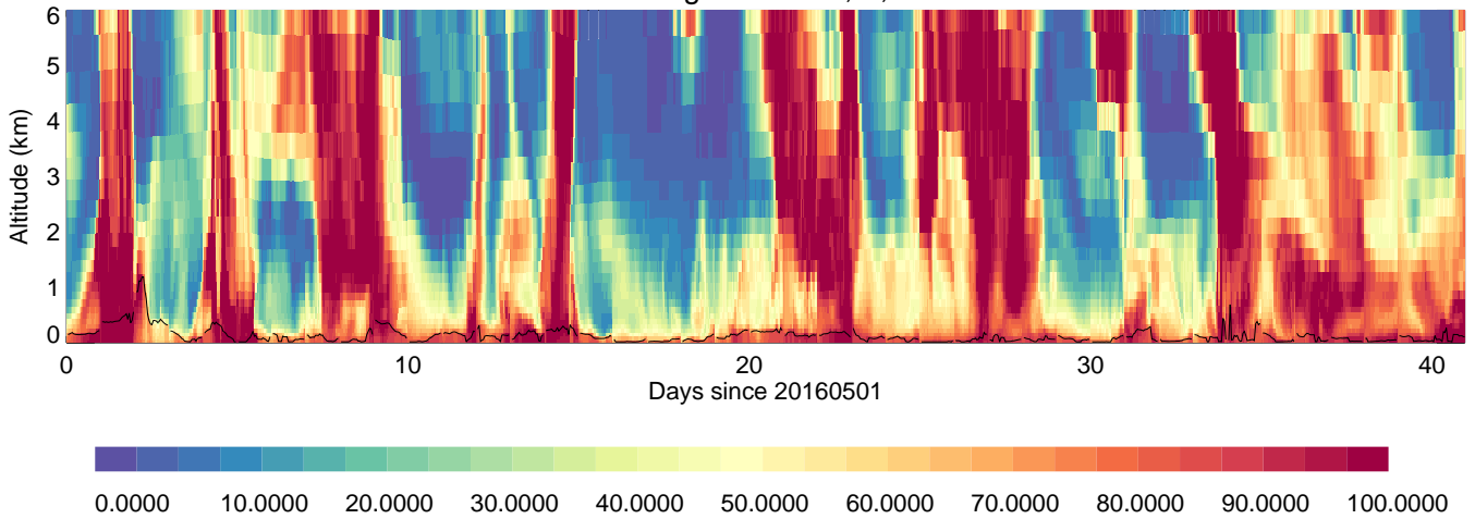
Gageocho: RH, %,
