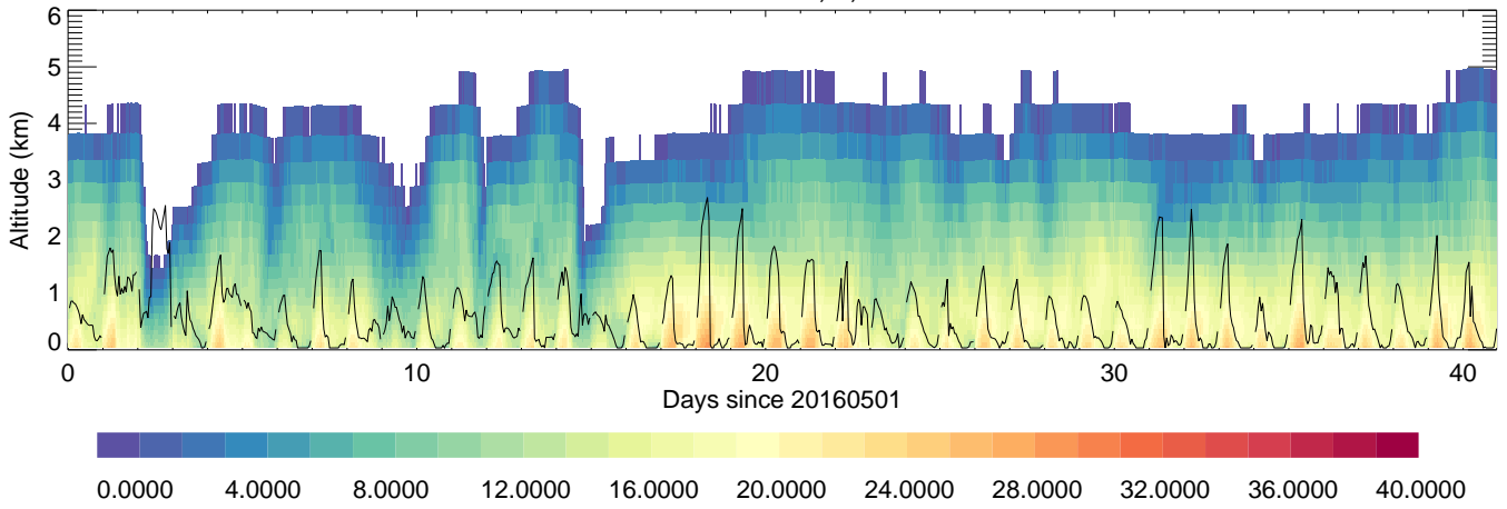
Osan: T,C,
