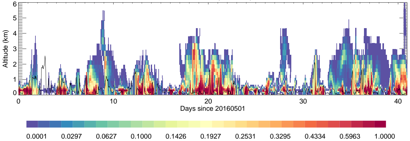
NIER: Point,unitless,
