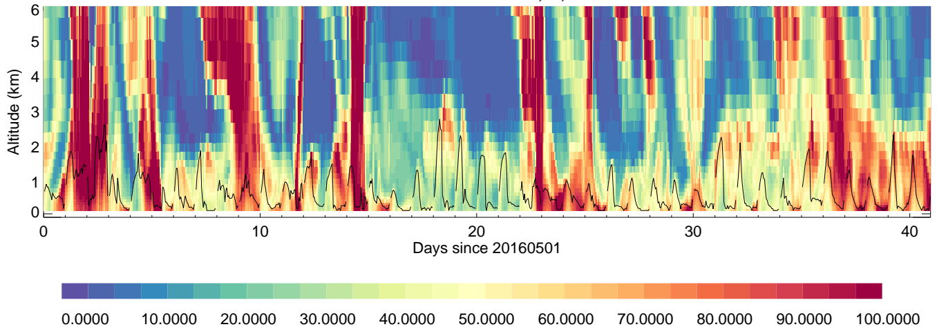
SeoulSNU: RH, %,
