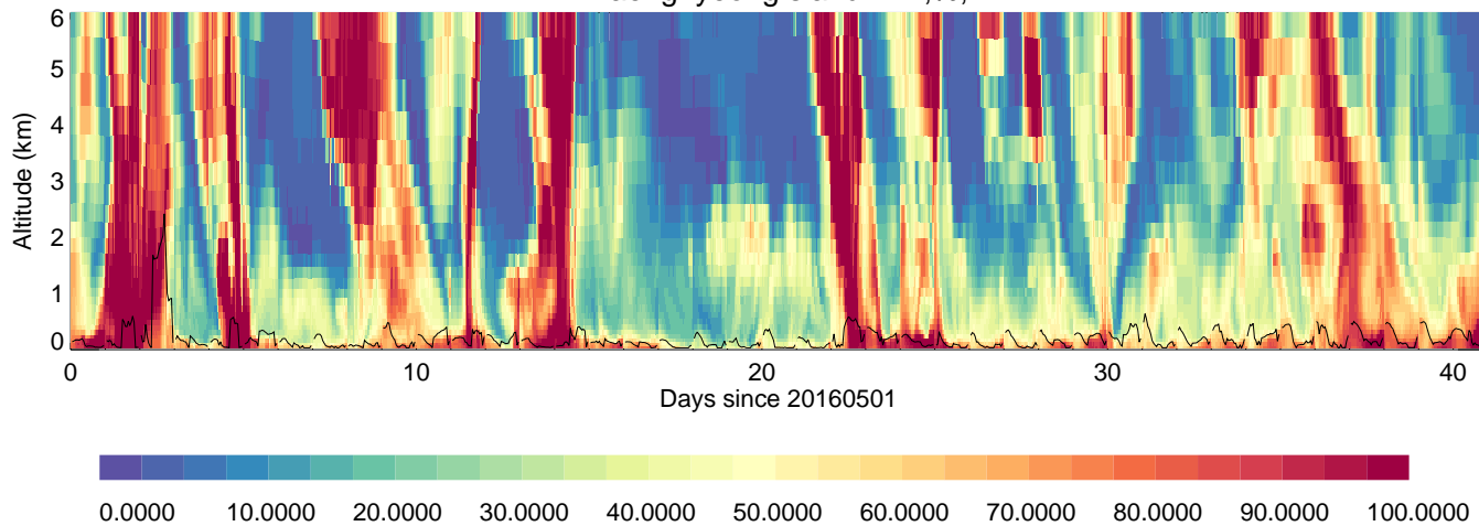
BaengnyeongIsland: RH,%,
