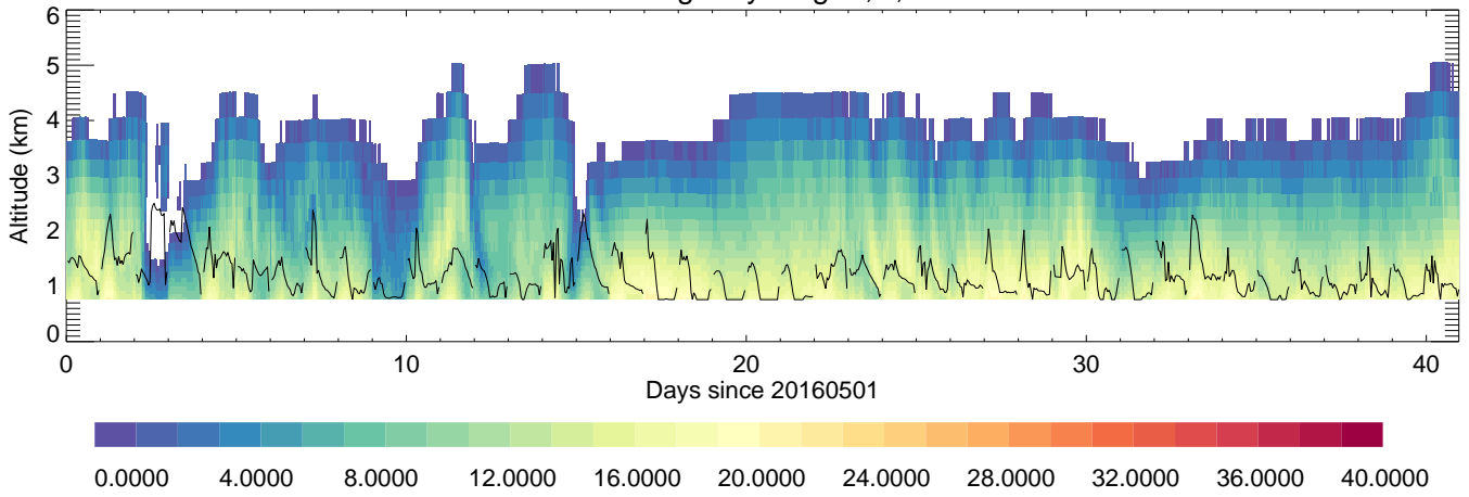
Daegwallyeong: T,C,
