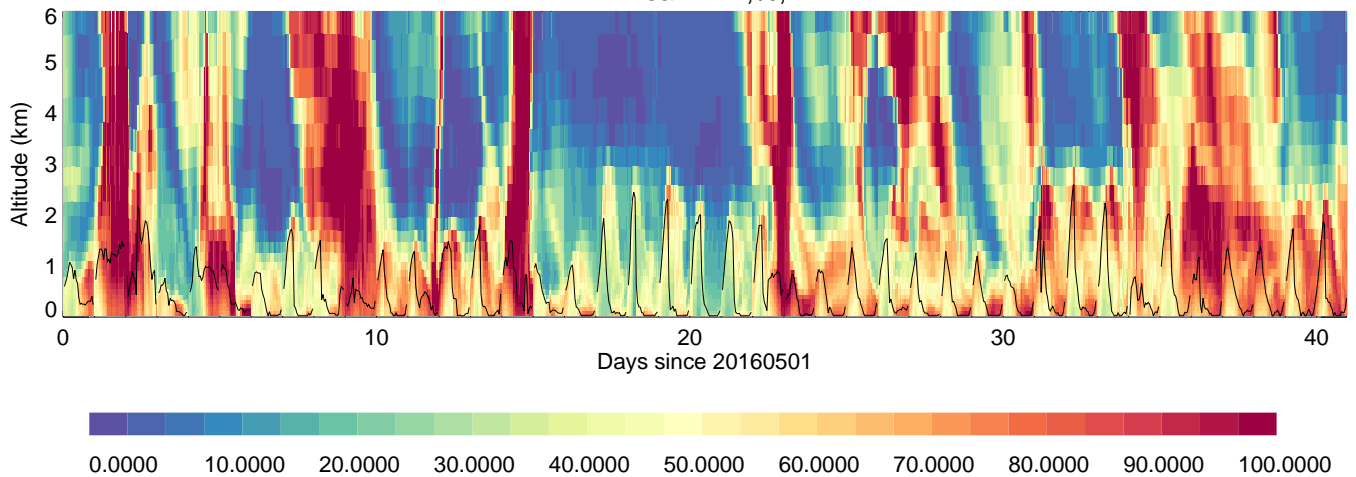
Iksan: RH, %,
