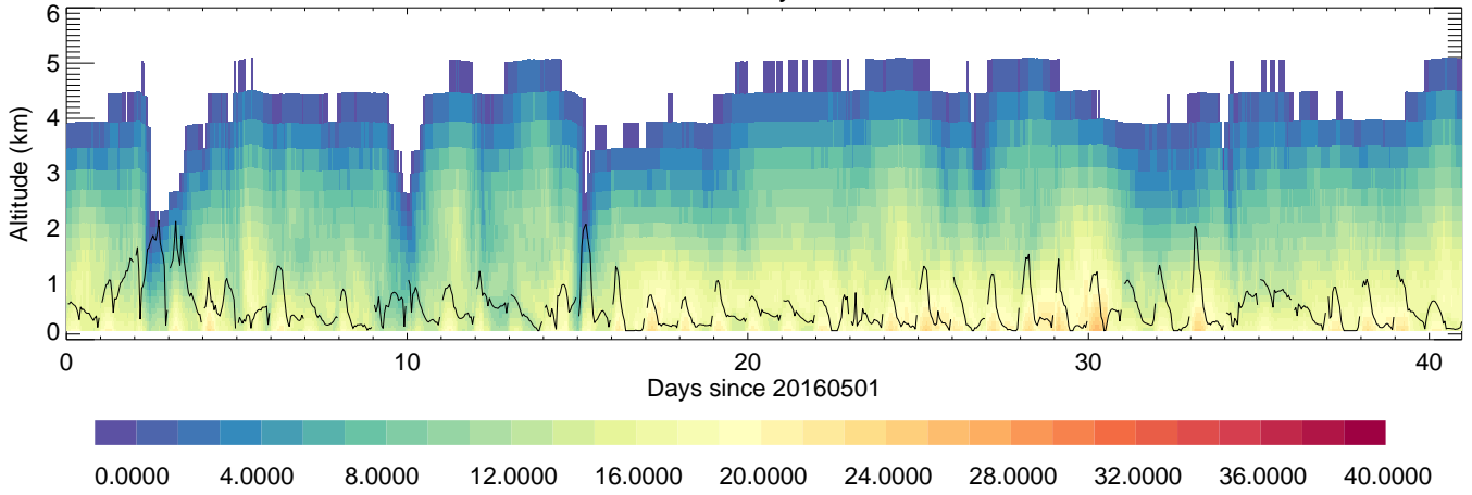
PusanUniversityBusan: T,C,
