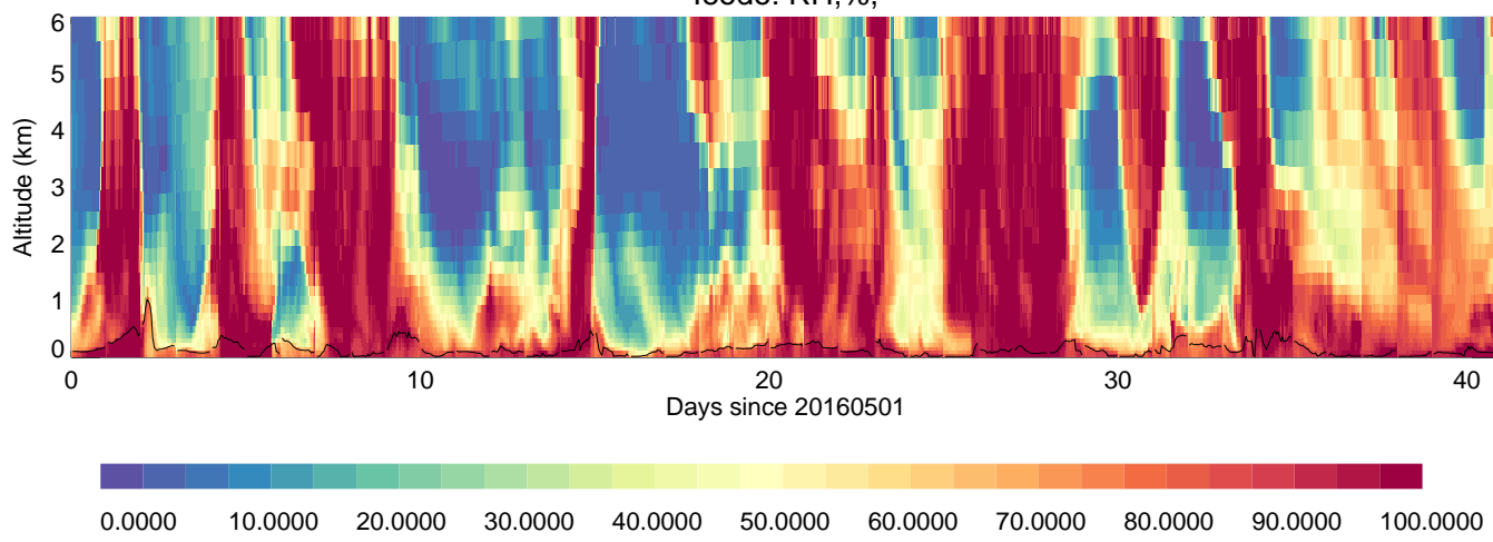
leodo: RH, %,
