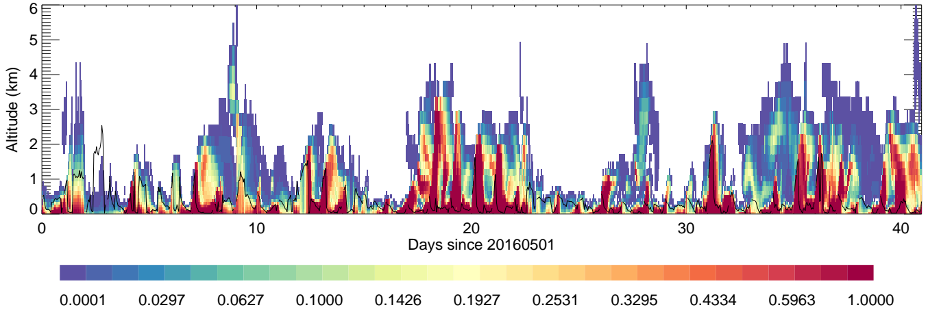
NIER: AreaMobile,unitless,
