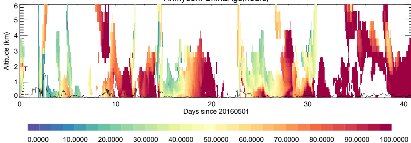
Anmyeon: RH, %,
