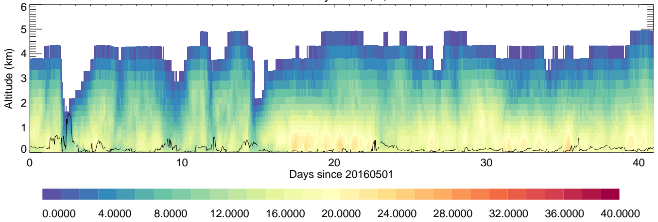
Anmyeon: T,C,
