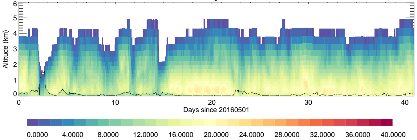
Socheongcho: T,C,
