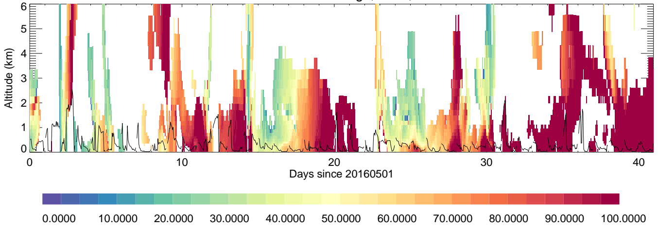
NIER: RH, %,
