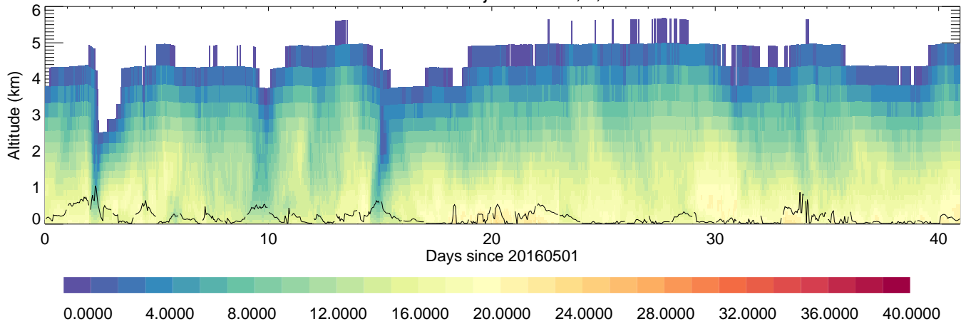
GosanJejulsland: T,C,
