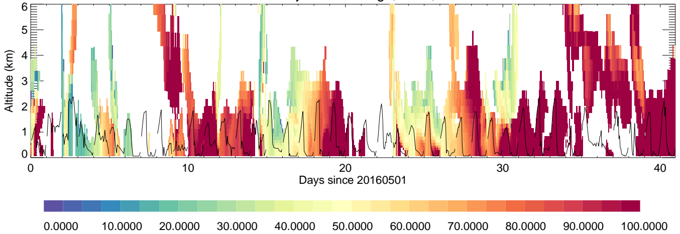
Daejeon: RH, %,
