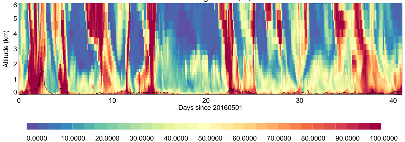
Socheongcho: RH, %,
