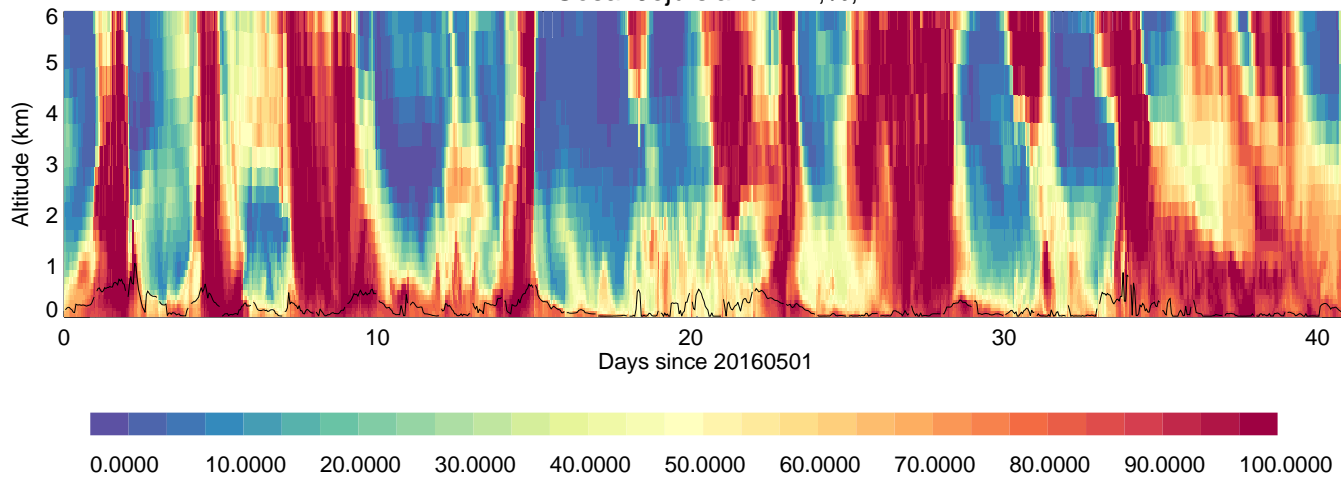
GosanJejulsland: RH, %,
