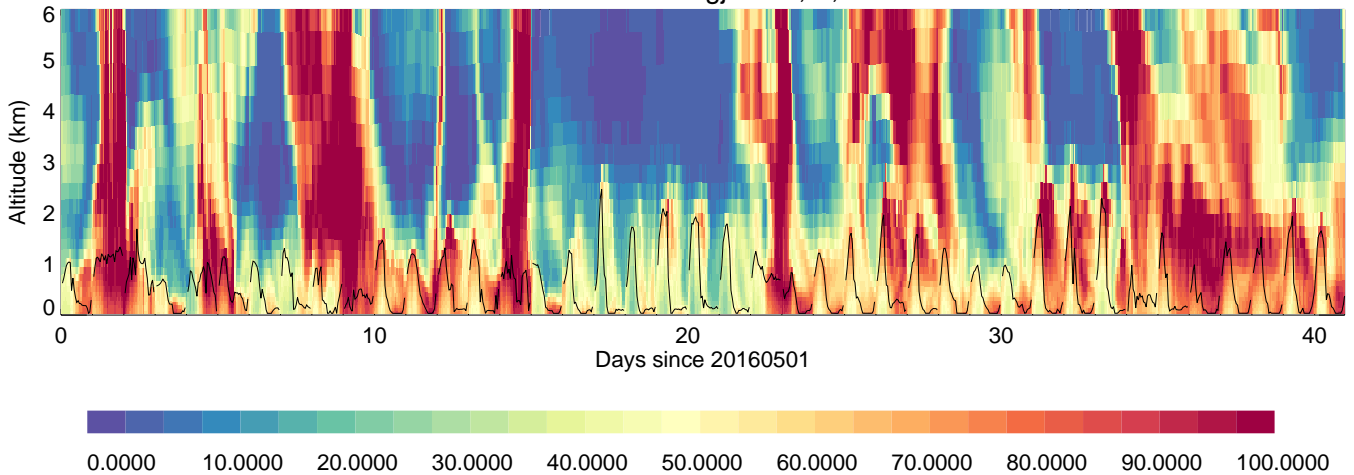
GISTGwangju: RH, %,
