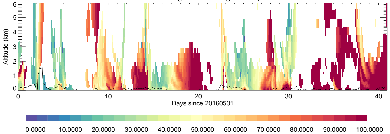
Socheongcho: RH, %,
