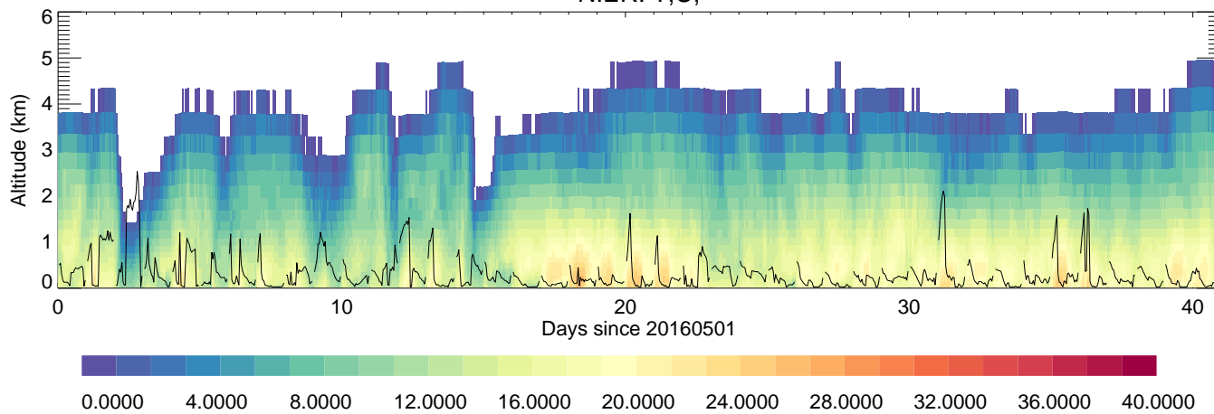
NIER: T,C,
