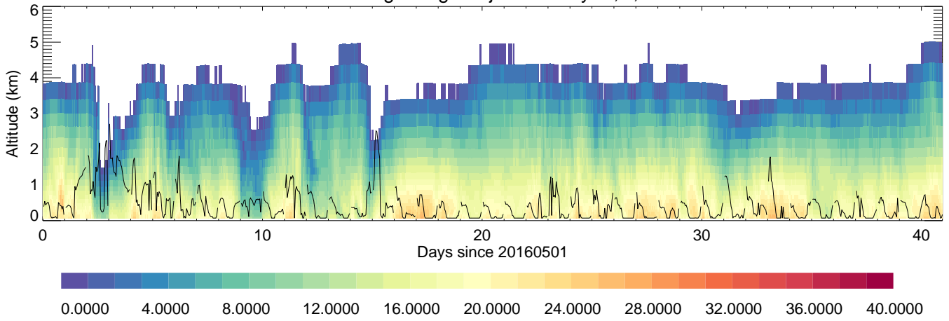
GangneungWonjuUniversity: T,C,
