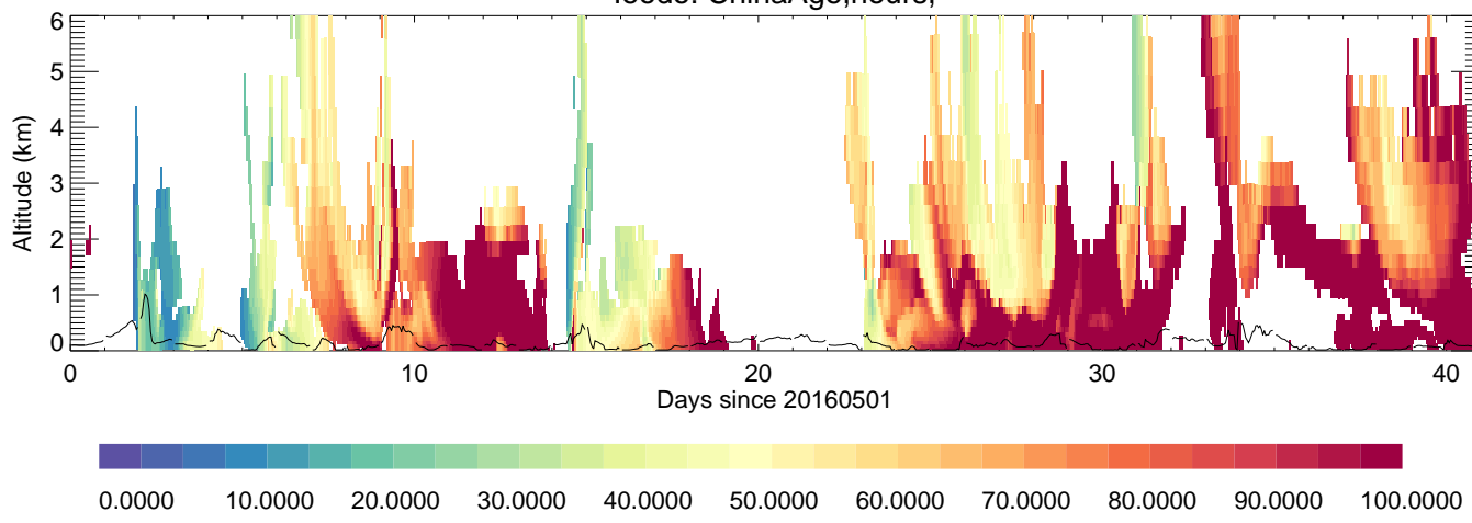
leodo: RH, %,
