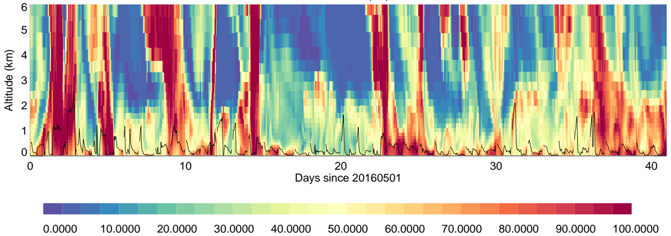
NIER: RH, %,
