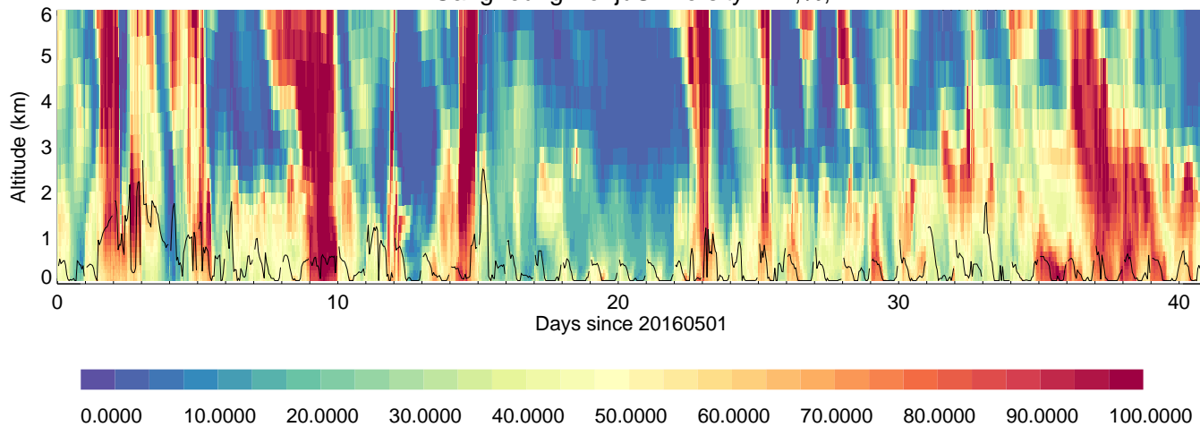
GangneungWonjuUniversity: RH,%,
