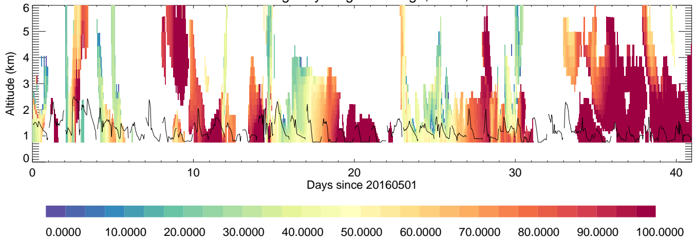
Daegwallyeong: RH, %,
