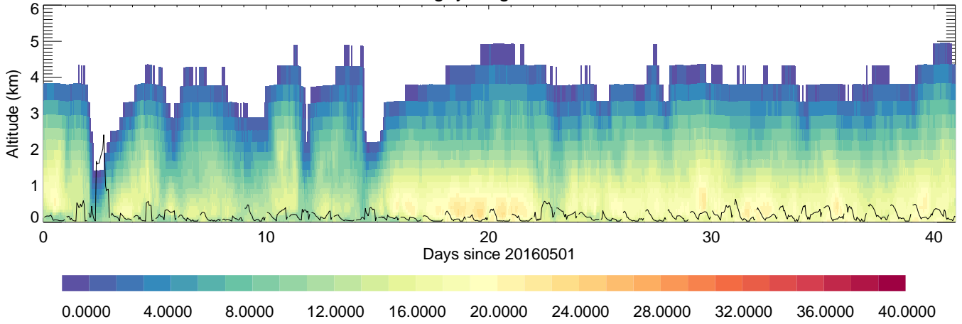
BaengnyeongIsland: T,C,
