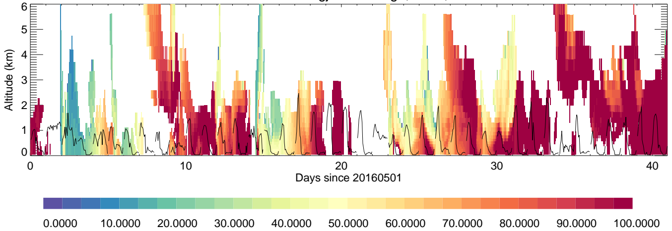
GISTGwangju: RH, %,
