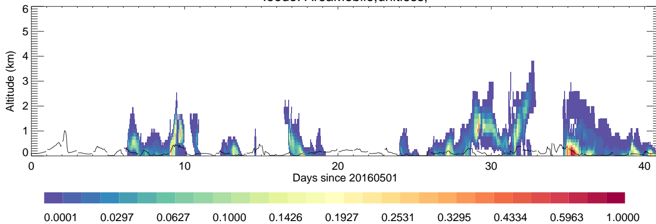
leodo: AreaMobile,unitless,
