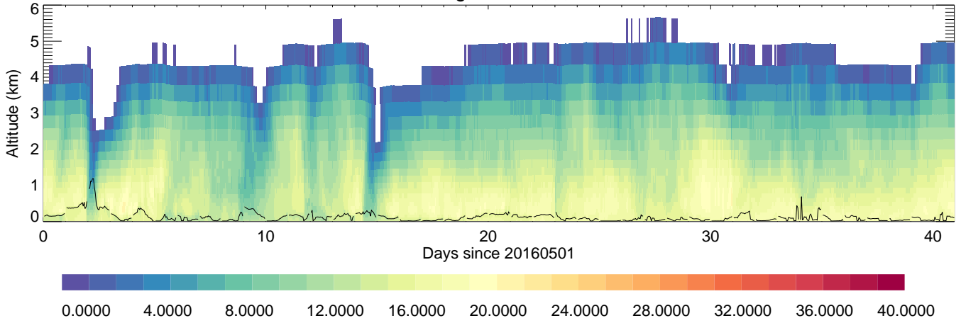
Gageocho: T,C,
