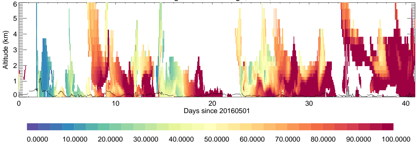
Gageocho: RH, %,
