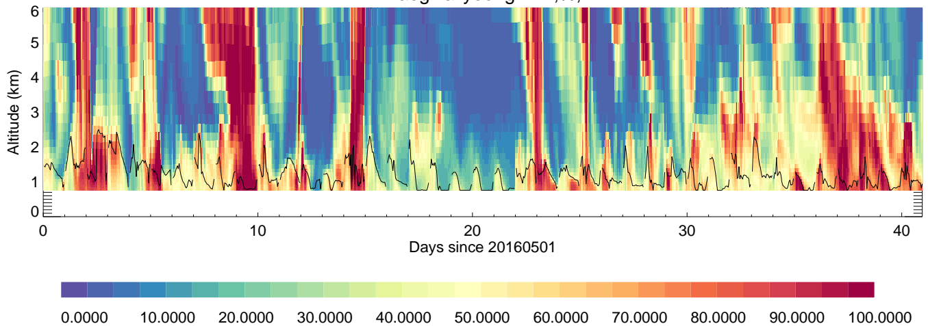
Daegwallyeong: RH, %,
