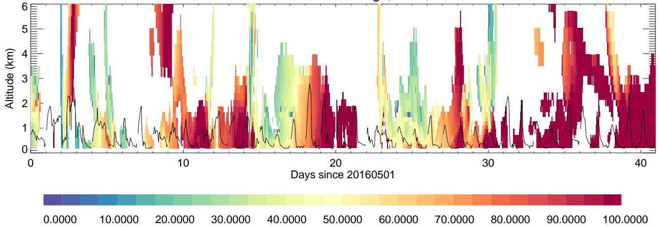
SeoulSNU: RH, %,
