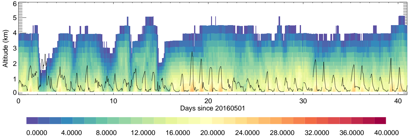
SeoulSNU: T,C,
