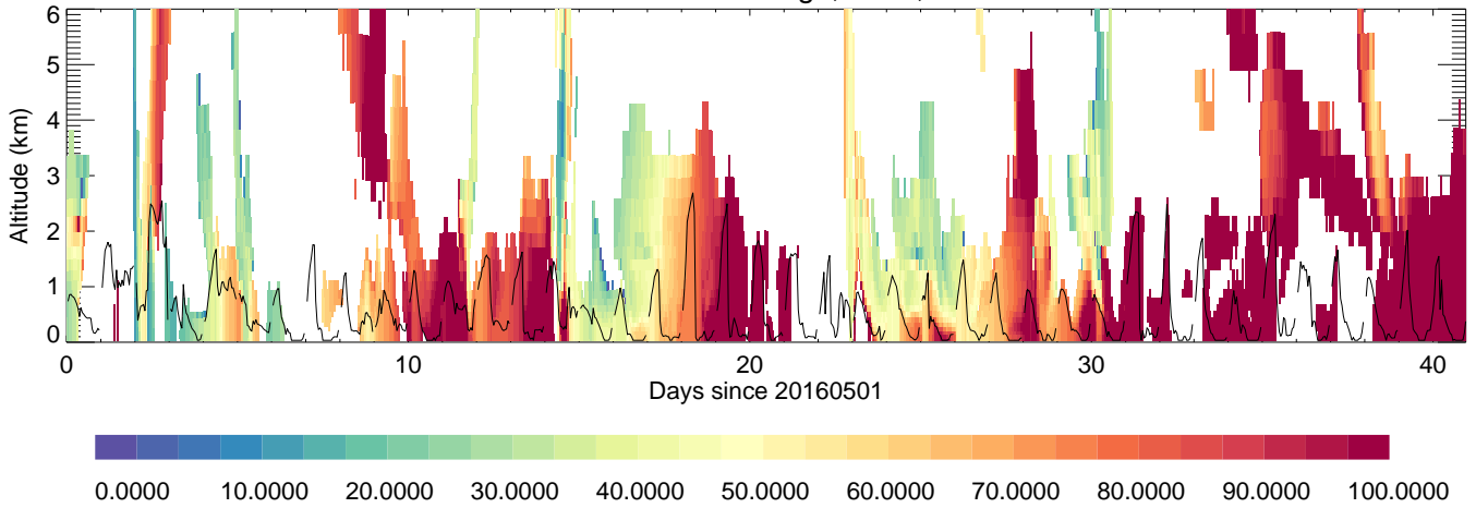
Osan: RH, %,
