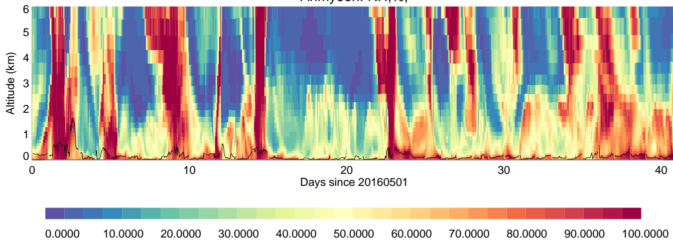
Anmyeon: RH, %,
