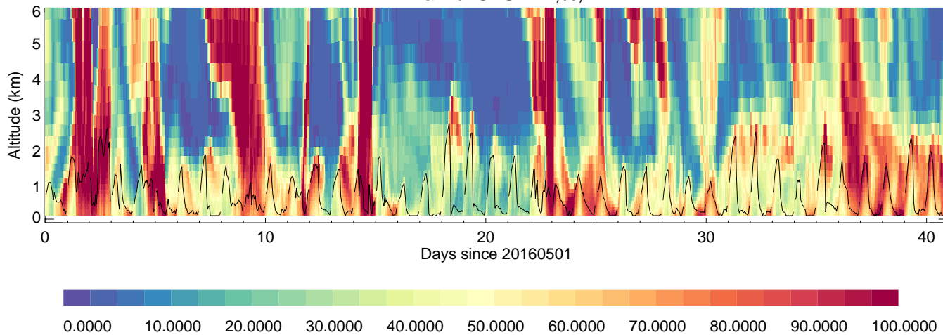
HankukUFS: RH, %,
