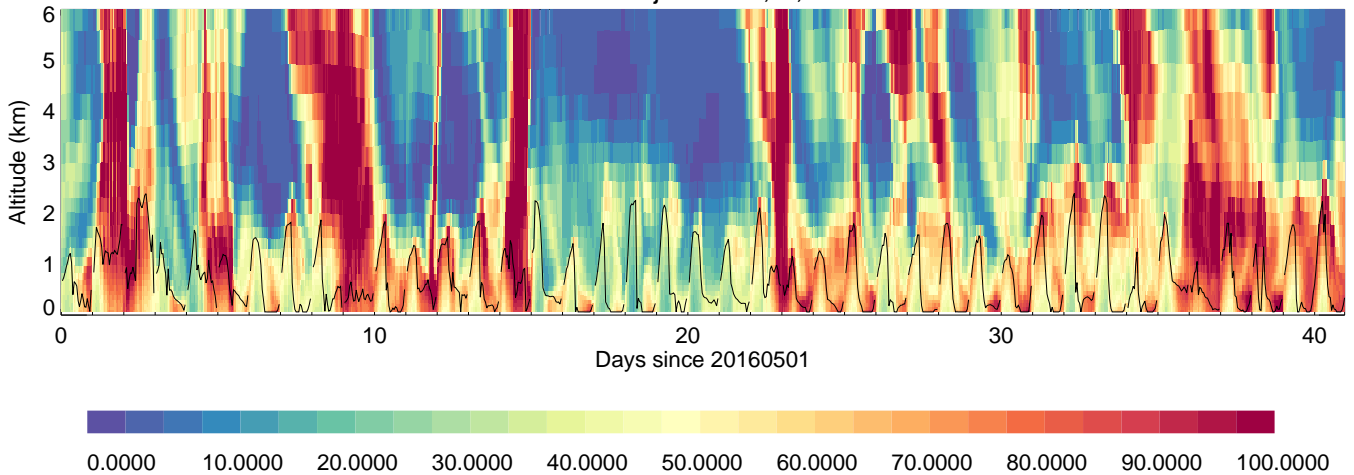
Daejeon: RH, %,
