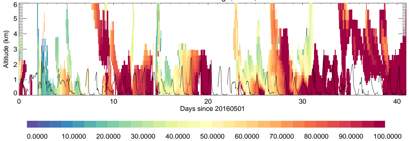
Iksan: RH, %,
