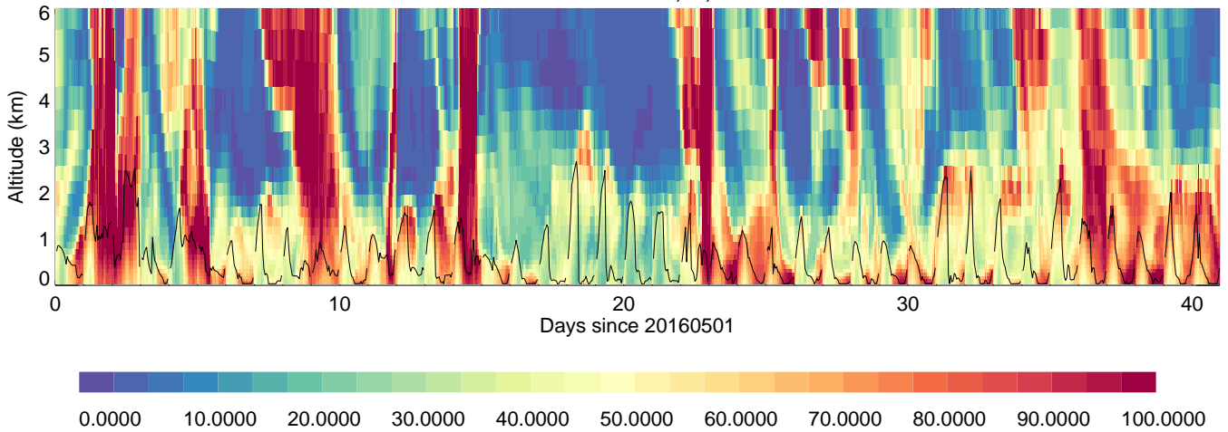
Osan: RH, %,
