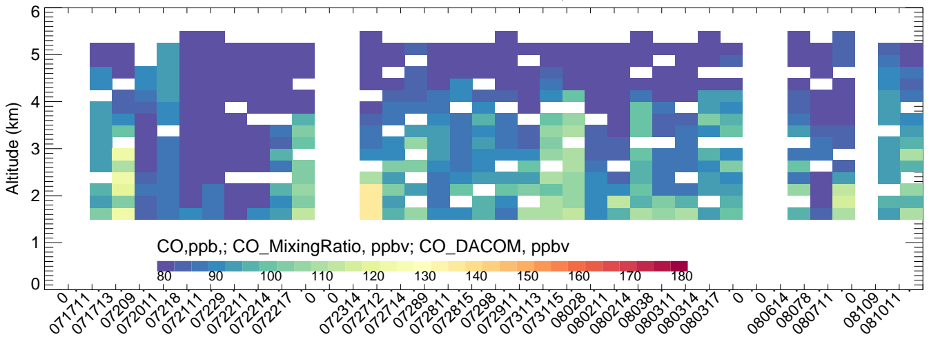
FortCollins CMAQ
