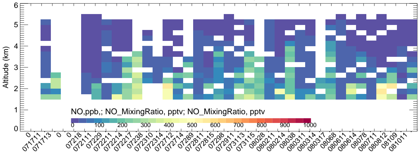
FortCollins CMAQ
