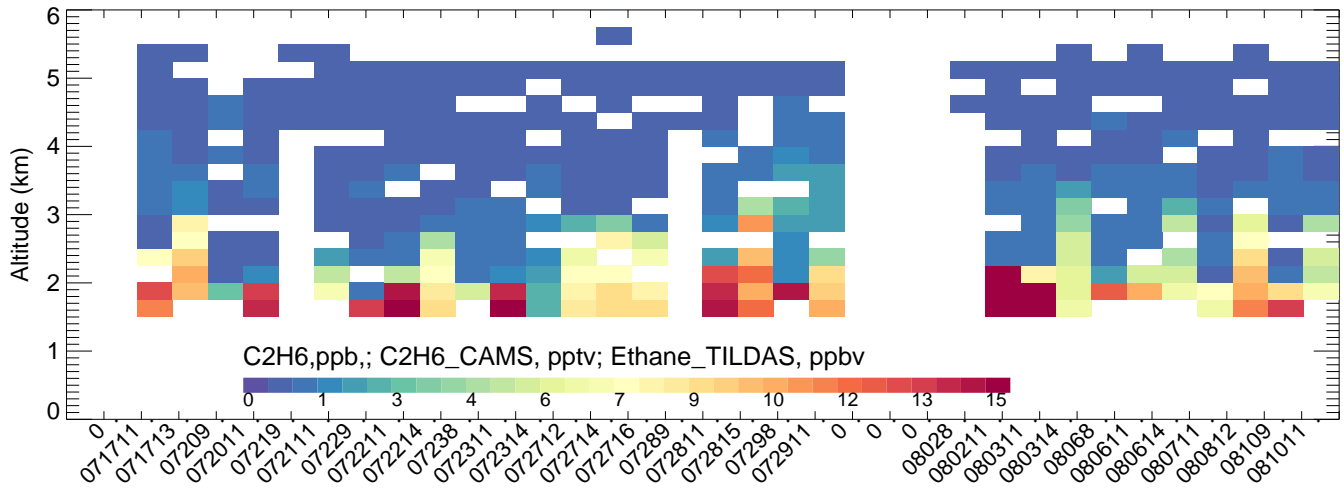
Platteville CMAQ
