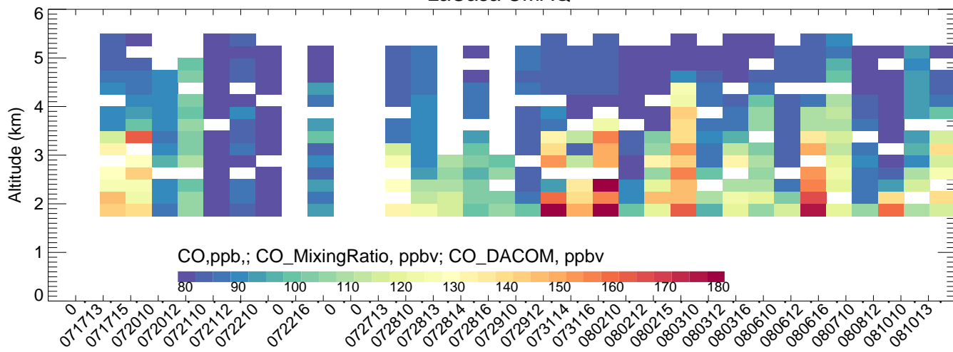
LaCasa CMAQ
