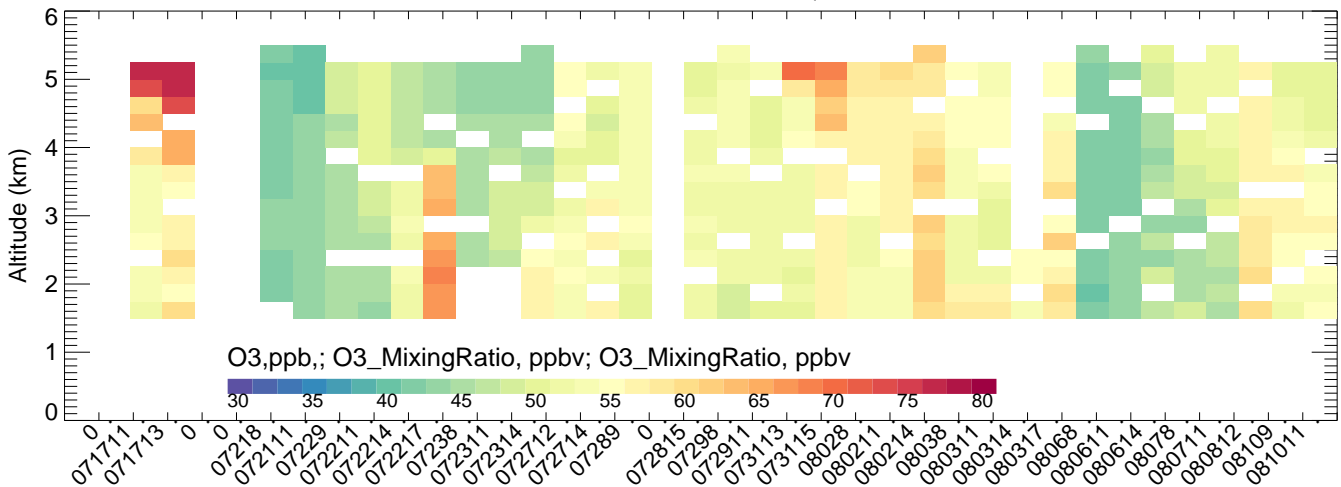
FortCollins CMAQ
