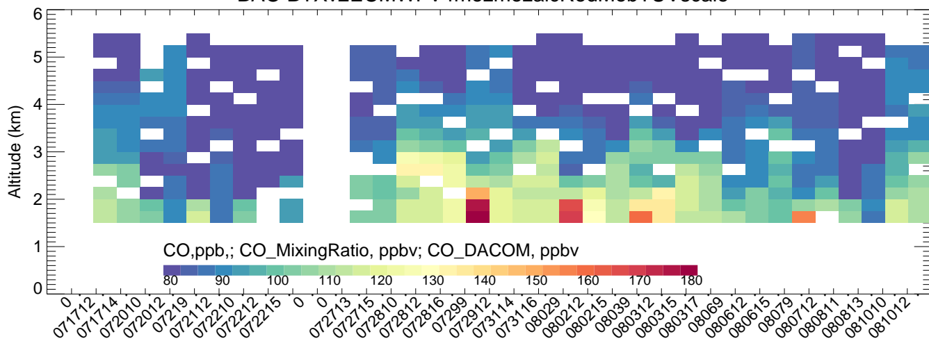
BAO CMAQ
