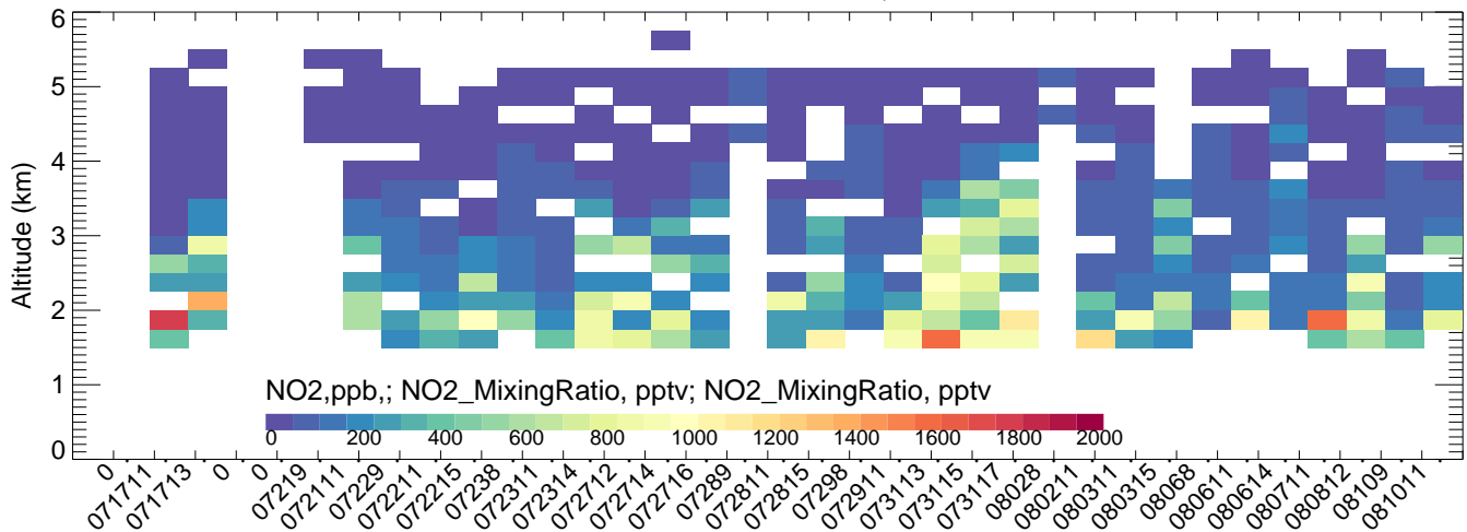
Platteville CMAQ
