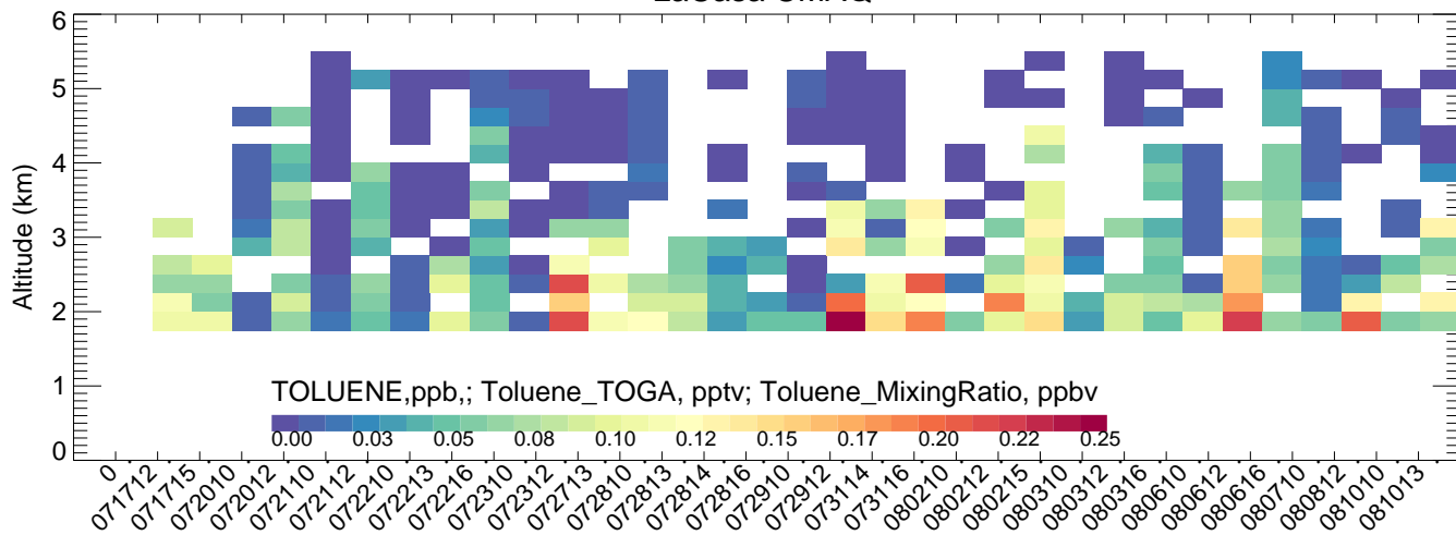
LaCasa CMAQ
