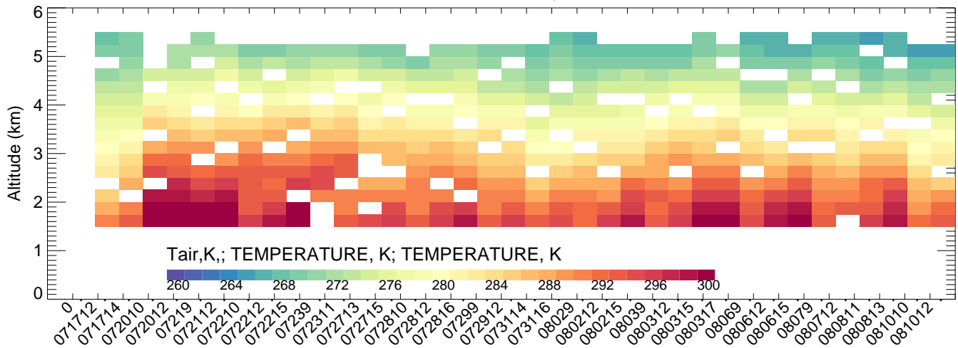
BAO CMAQ
