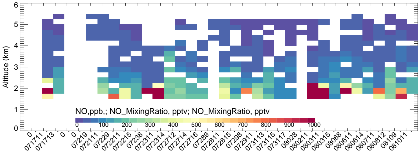
Platteville CMAQ
