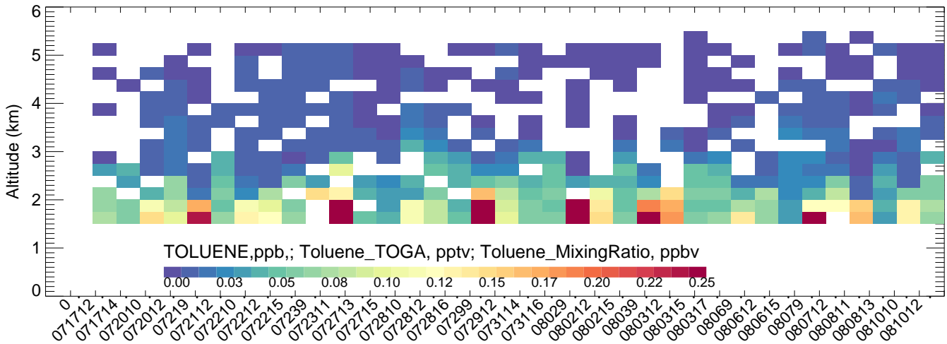
BAO CMAQ
