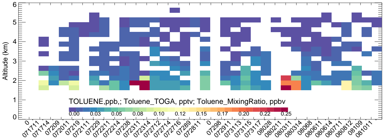
Platteville CMAQ
