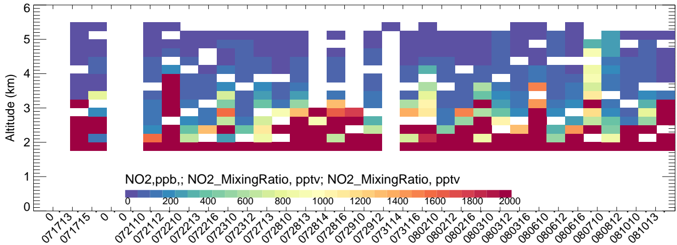
LaCasa CMAQ
