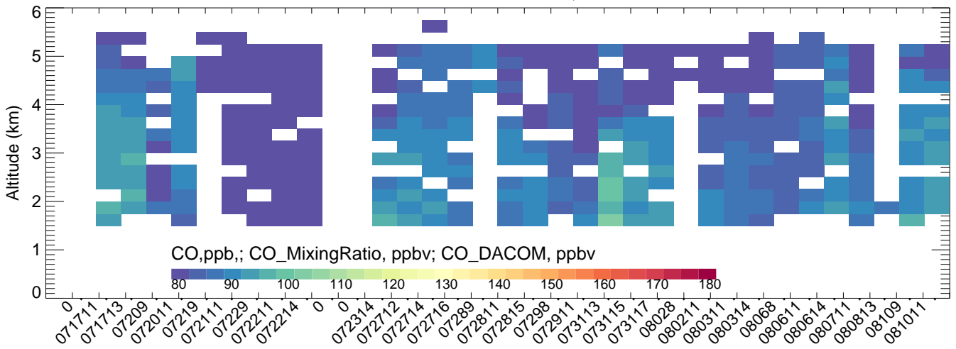
Platteville CMAQ
