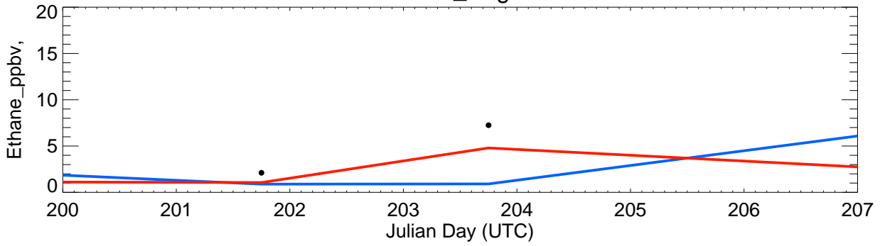
VOCCAN_Sugarloaf
