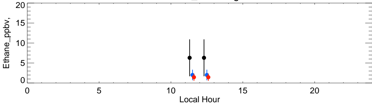
VOCCAN_Lost-Angels
