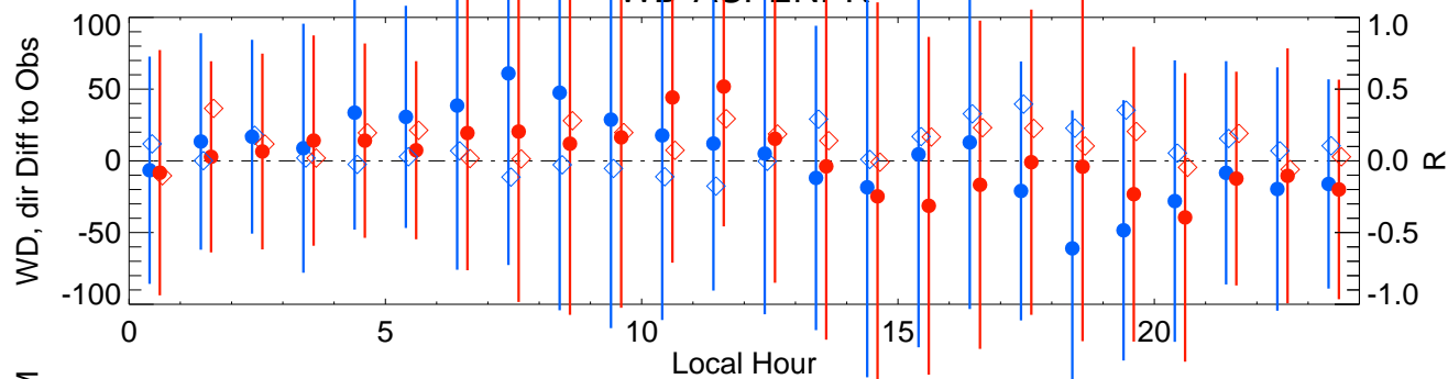
WD-ASPENPK
