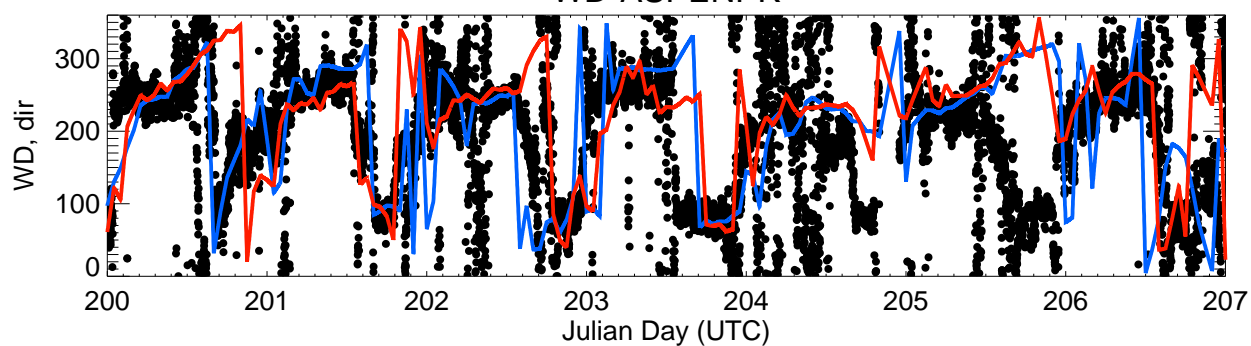
WD-ASPENPK
