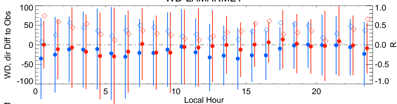
WD-LAMARMET
