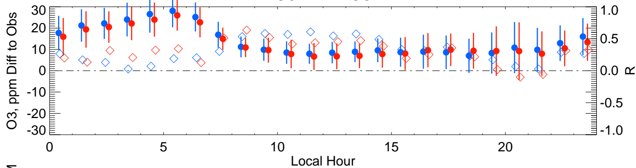
O3-RIFLEO3
