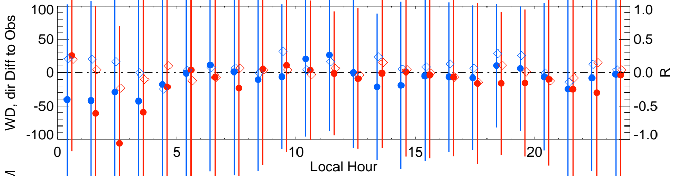
WD-FTC-CSU
