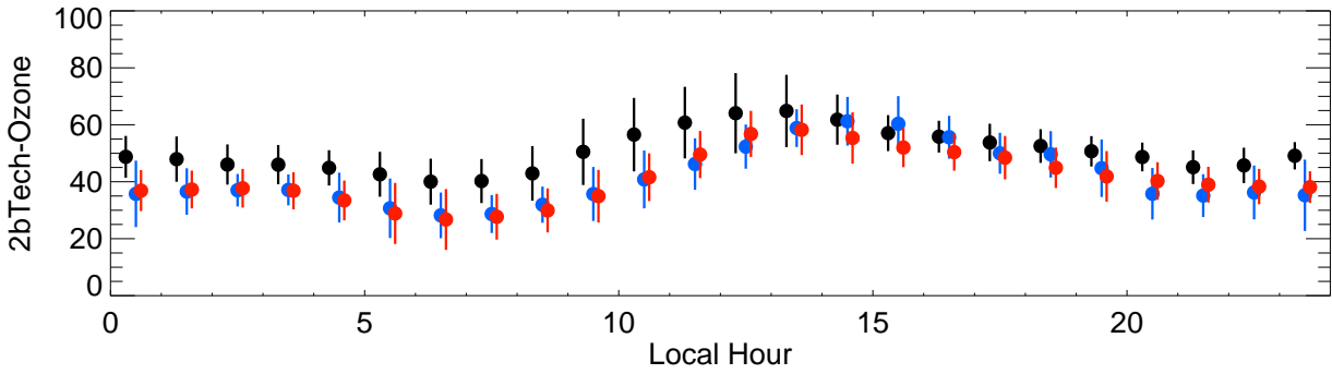
2bTech-Ozone-DanielsPark
