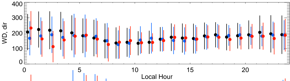
WD-FTC-CSU
