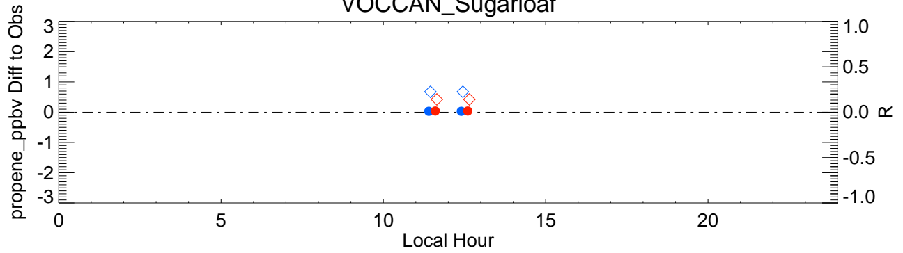
VOCCAN_Sugarloaf
