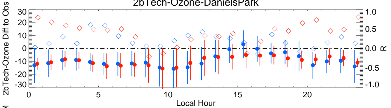
2bTech-Ozone-DanielsPark
