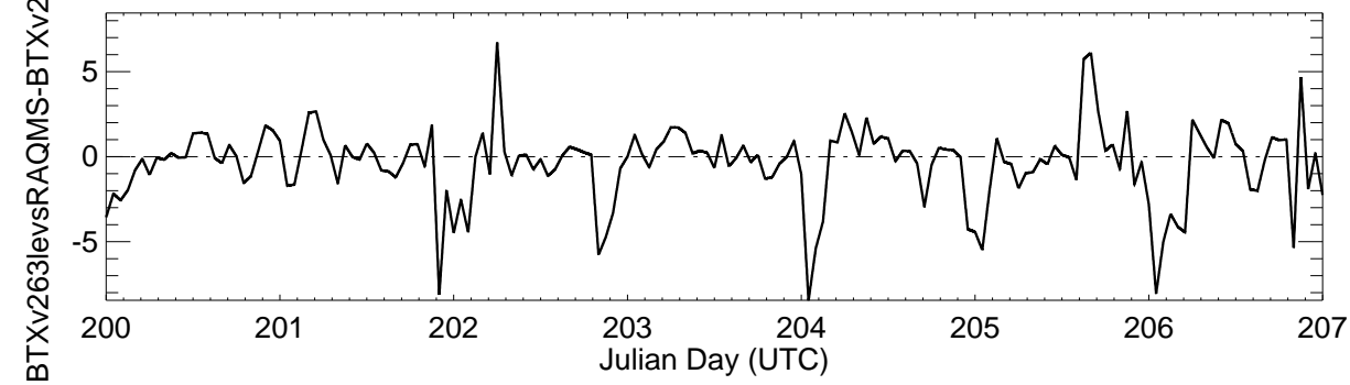
WS-LACASA
