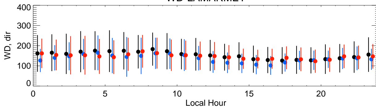
WD-LAMARMET
