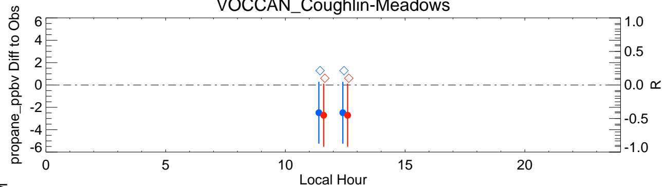
VOCCAN_Coughlin-Meadows
