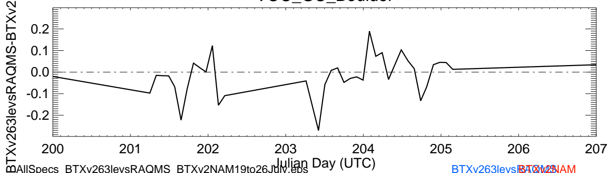
VOC_GC_Boulder
