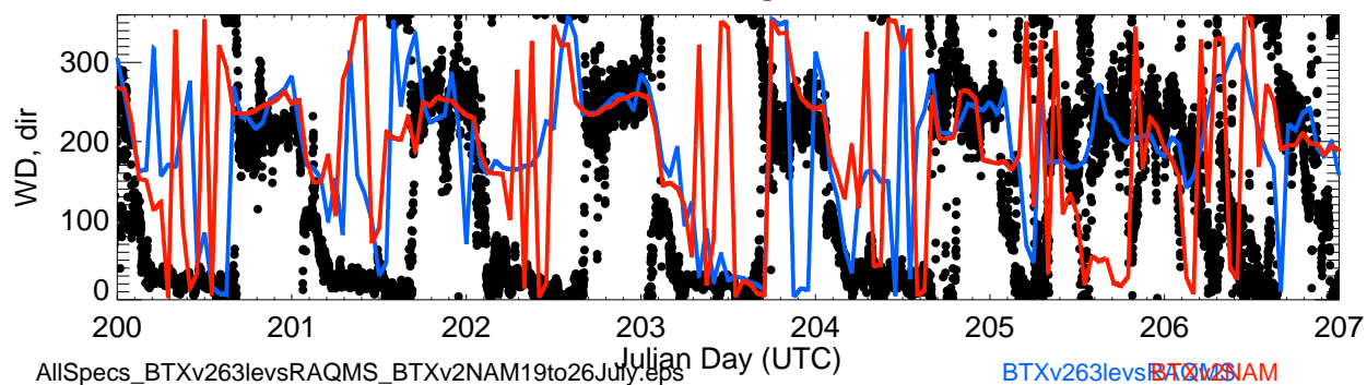
WD-PALISADE
