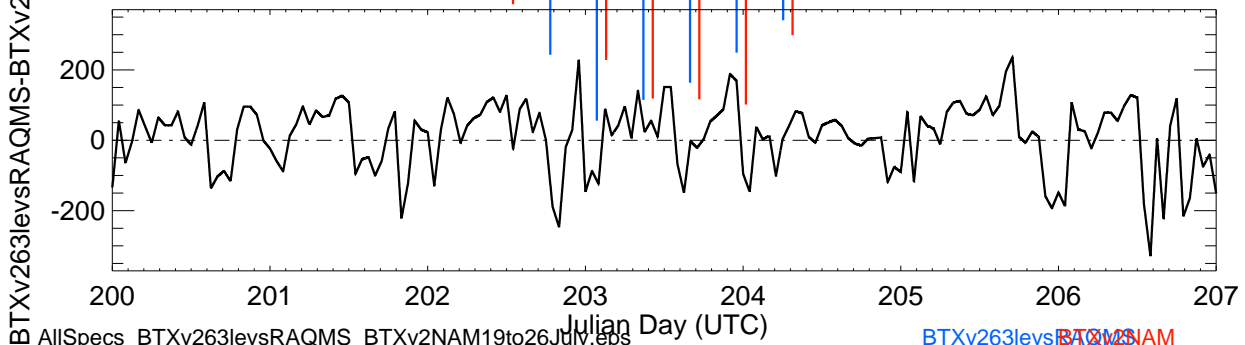
WD-CHATPARK
