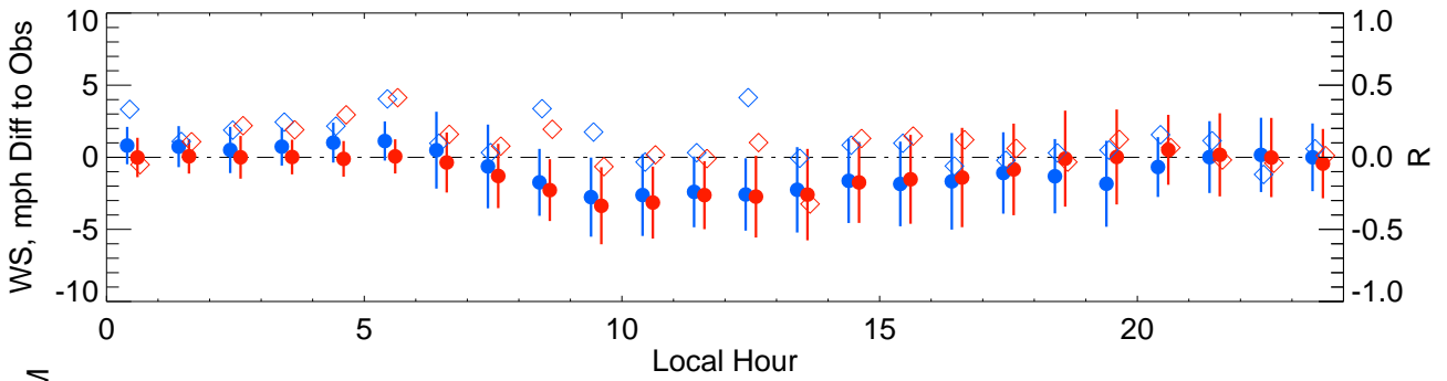
WS-ARVADA
