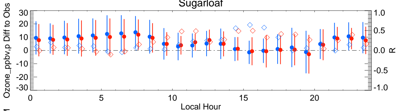
Sugarloaf
