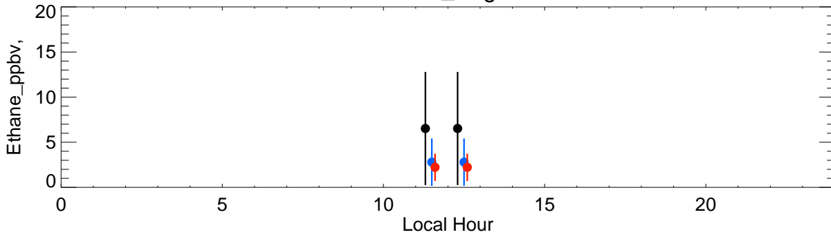
VOCCAN_Sugarloaf
