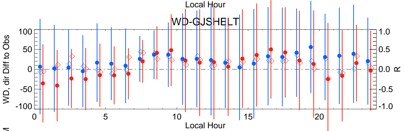
WD-GJSHELT
