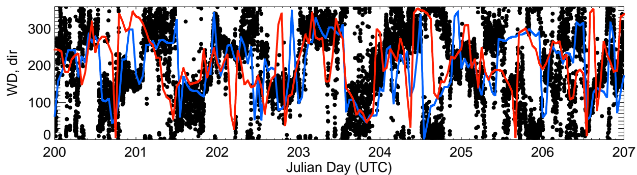
WD-ARVADA
