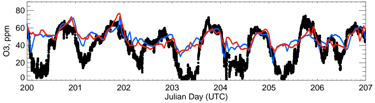
O3-ACADEMY
