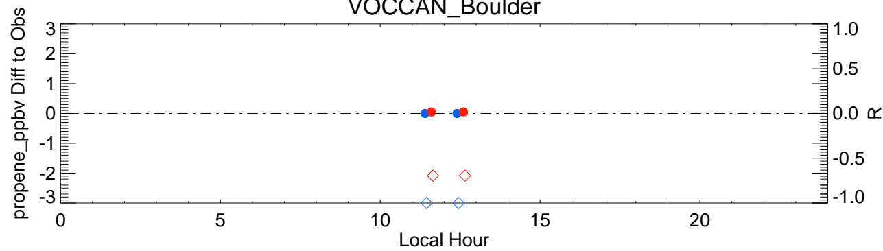
VOCCAN_Boulder
