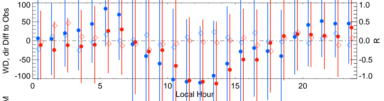
WD-CHATPARK
