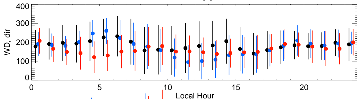
WD-ALSUP
