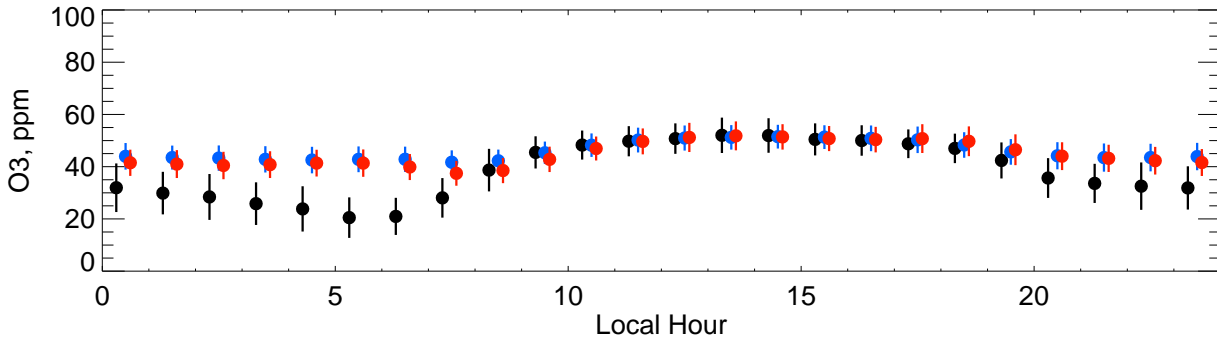
O3-CORTEZ
