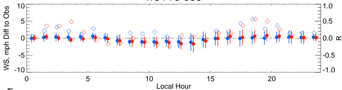
WS-FTC-CSU
