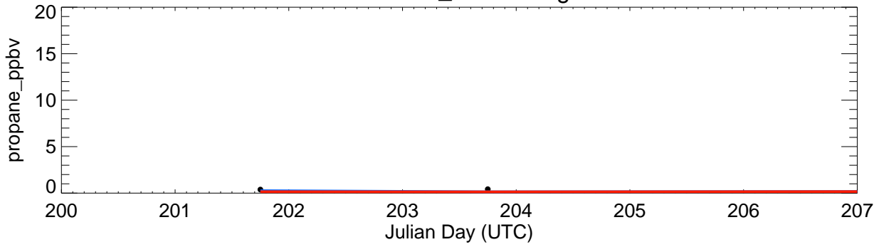
VOCCAN_Niwot-Ridge
