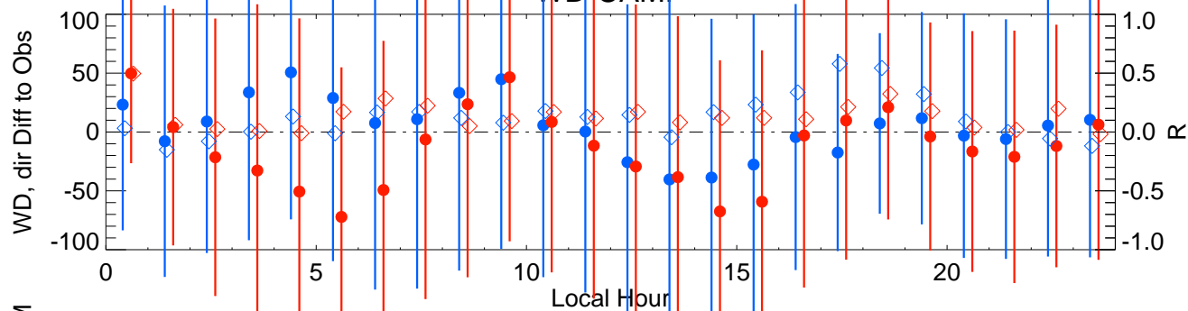
WD-CAMP
