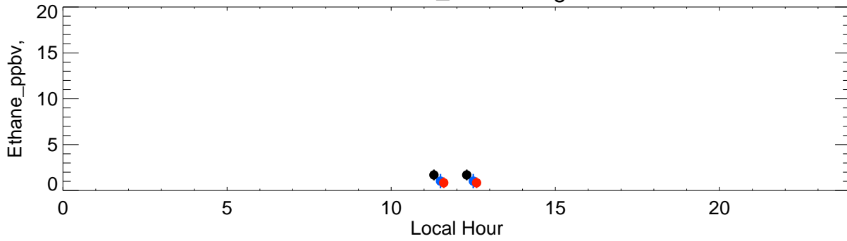
VOCCAN_Niwot-Ridge
