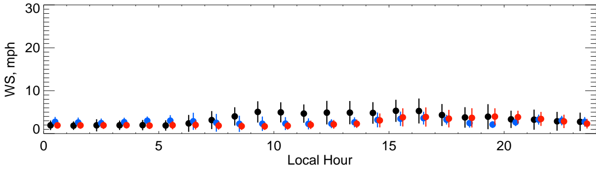
WS-ARVADA
