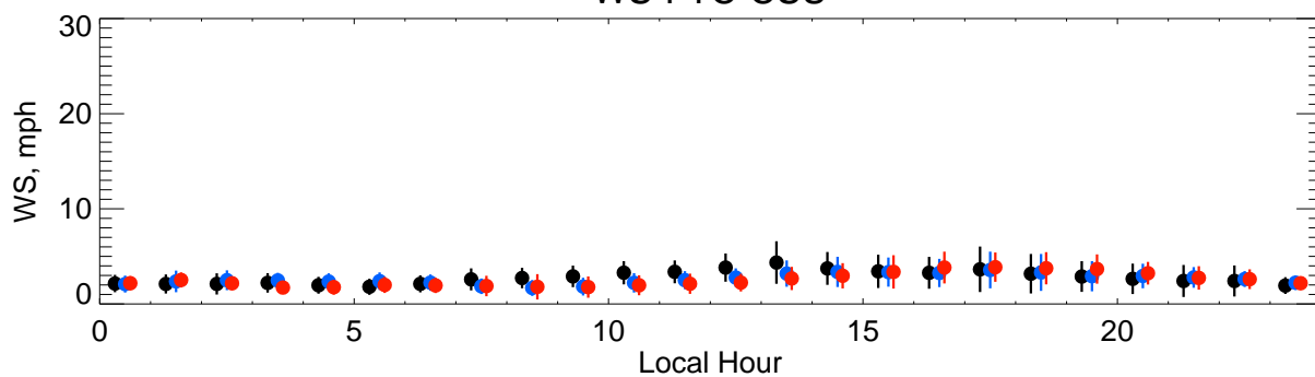
WS-FTC-CSU
