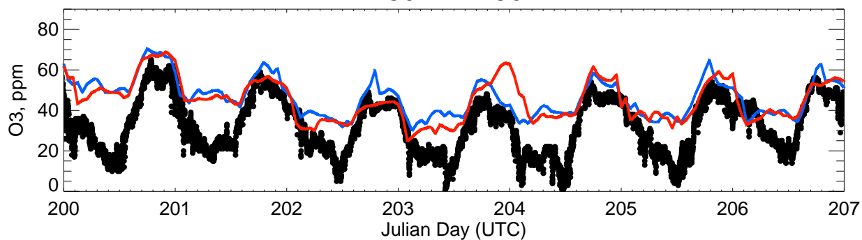
O3-RIFLEO3
