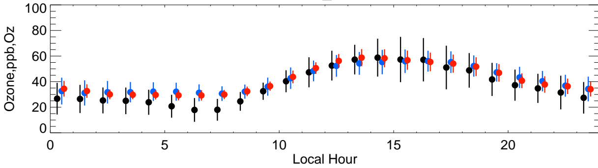
-FortCollins-CSU_GROUND-Other
