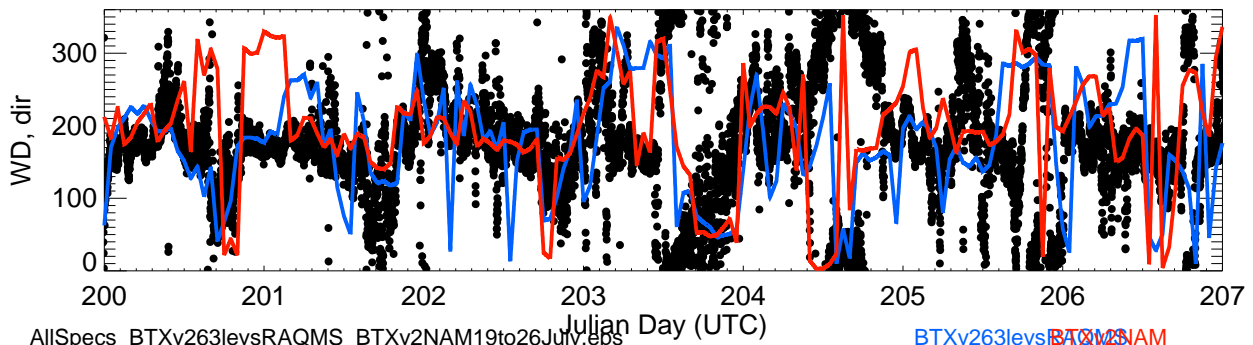
WD-I25-DENVER
