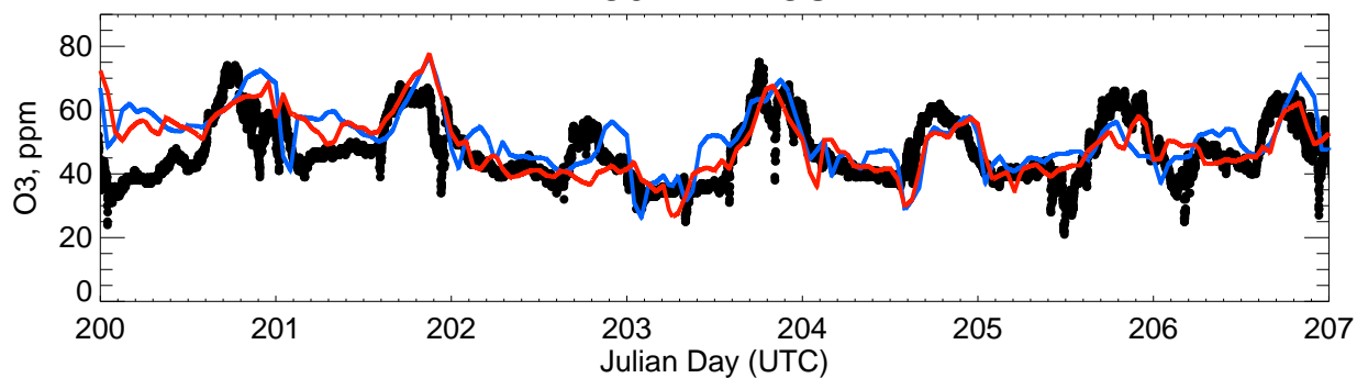
O3-MANITOU
