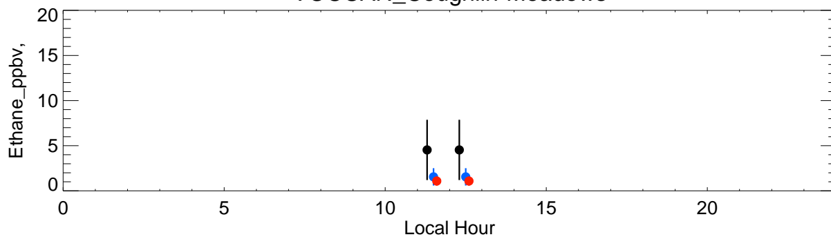
VOCCAN_Coughlin-Meadows
