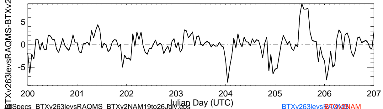
WS-ARVADA
