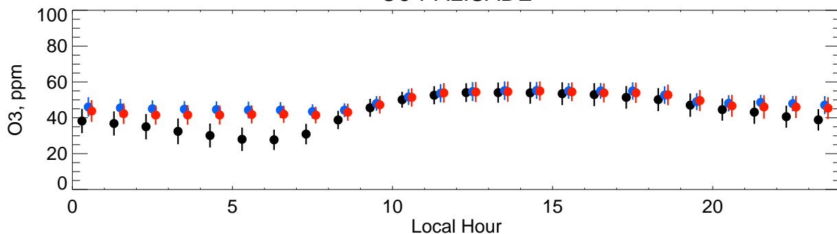
O3-PALISADE
