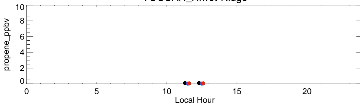
VOCCAN_Niwot-Ridge
