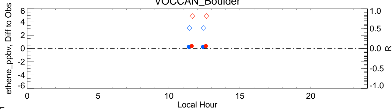
VOCCAN_Boulder
