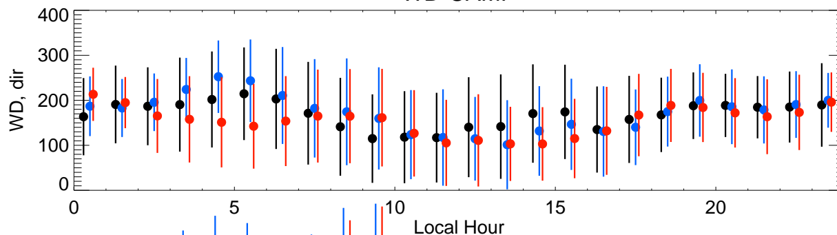
WD-CAMP
