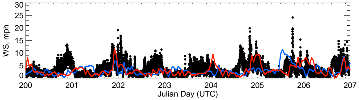
WS-ARVADA
