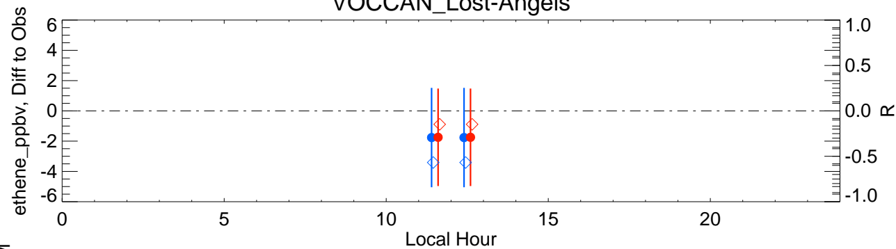
VOCCAN_Lost-Angels
