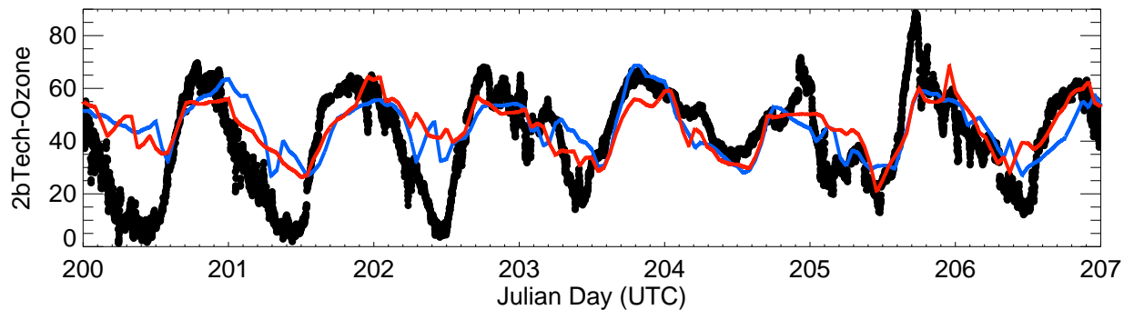
2bTech-Ozone-JacksonLake
