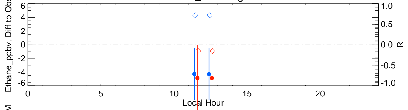
VOCCAN_Lost-Angels
