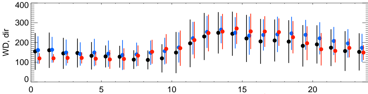
WD-GJSHELT
