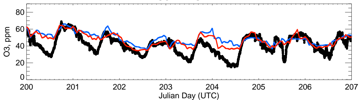
O3-PALISADE
