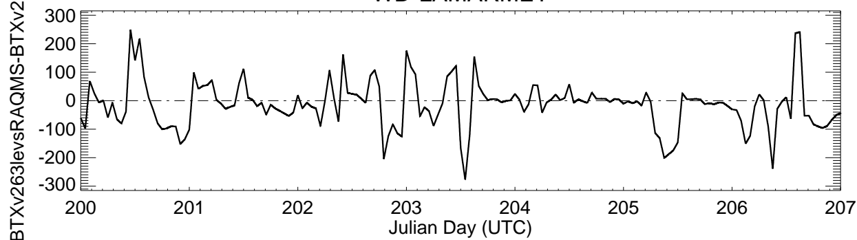
WD-PALISADE
