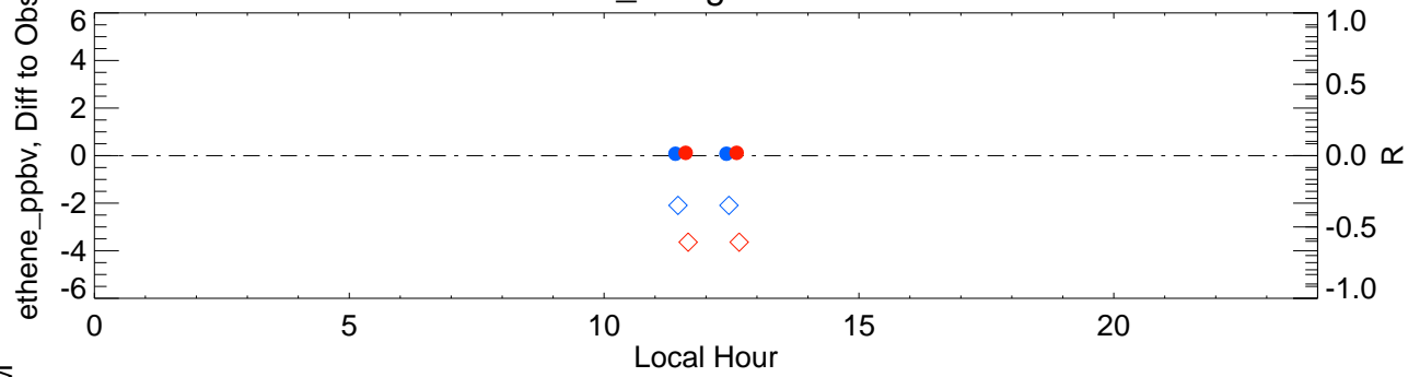
VOCCAN_Coughlin-Meadows
