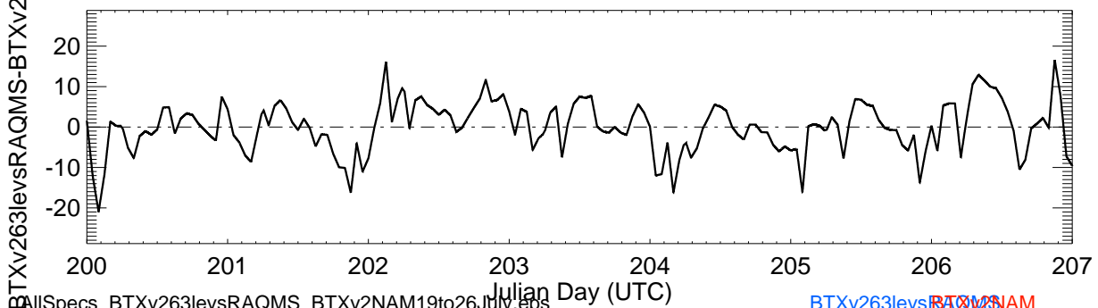
O3-ACADEMY
