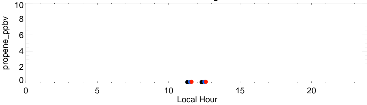
VOCCAN_Sugarloaf
