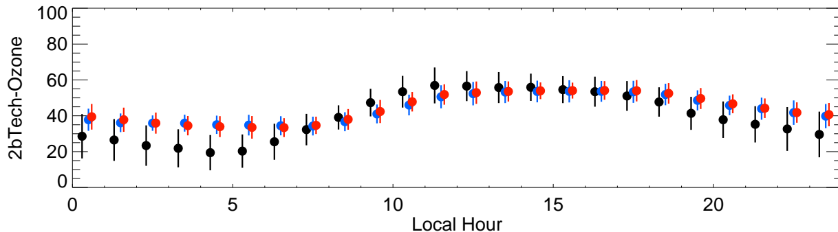
2bTech-Ozone-JacksonLake
