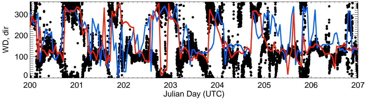
WD-GJSHELT
