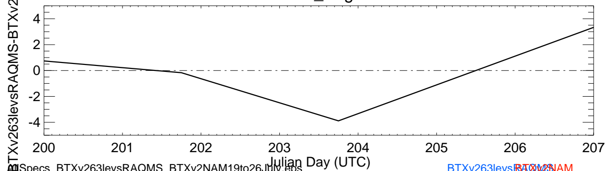
VOCCAN_Sugarloaf
