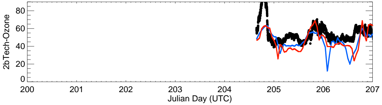
2bTech-Ozone-DanielsPark
