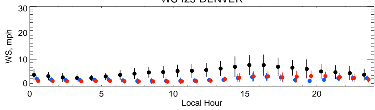
WS-I25-DENVER
