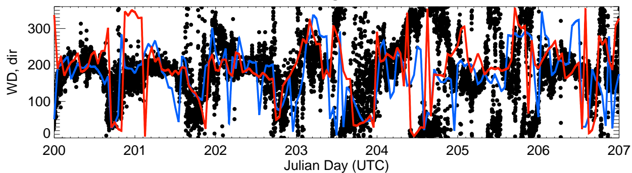
WD-CAMP
