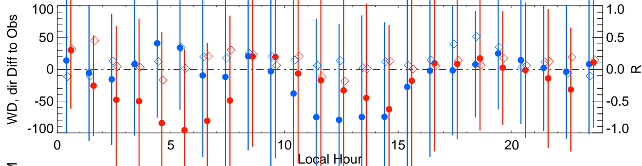
WD-ALSUP
