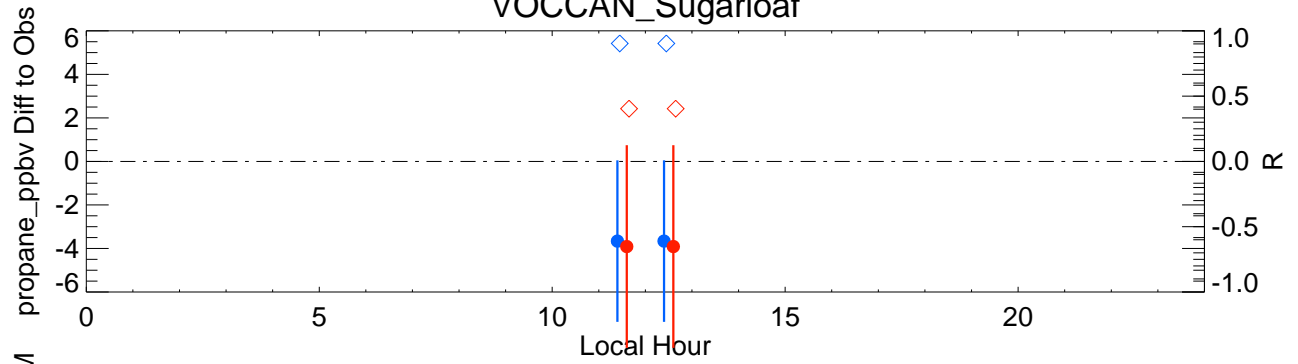
VOCCAN_Sugarloaf
