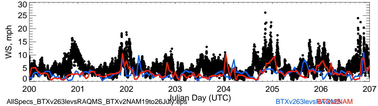
WS-LACASA
